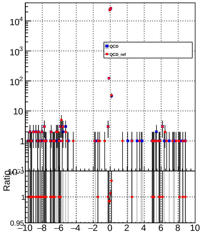
METUnc_MuonEnDown
