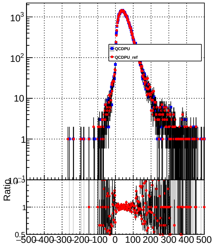
METDifference_GenMETTrue
