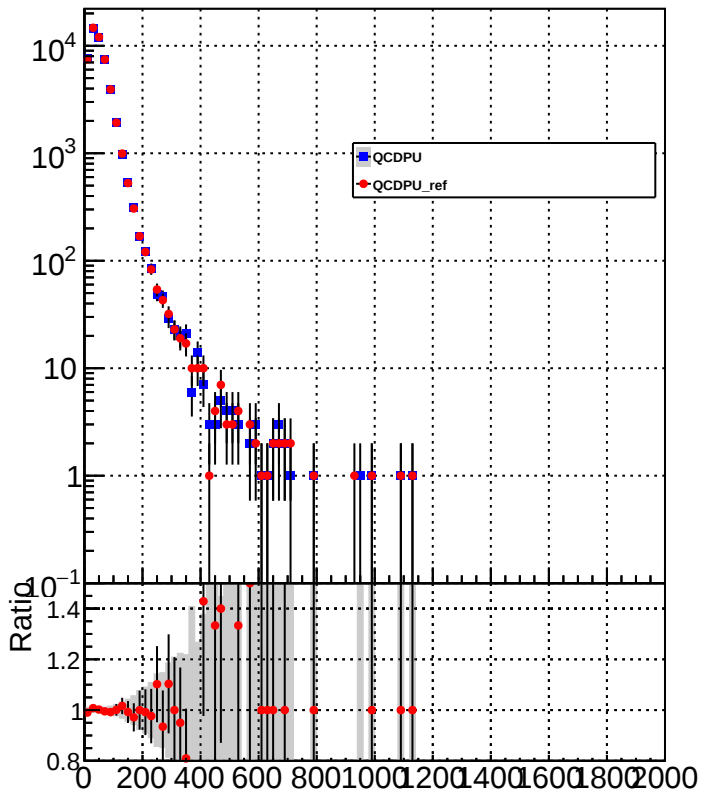
MET (20 GeV binning)
