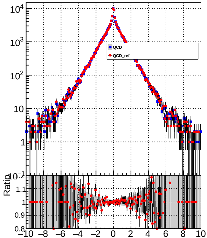
METUnc_UnclusteredEnDown
