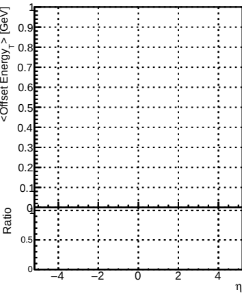
p_offset_eta_npv26_lep
