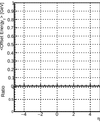
p_offset_eta_npv26_chm
