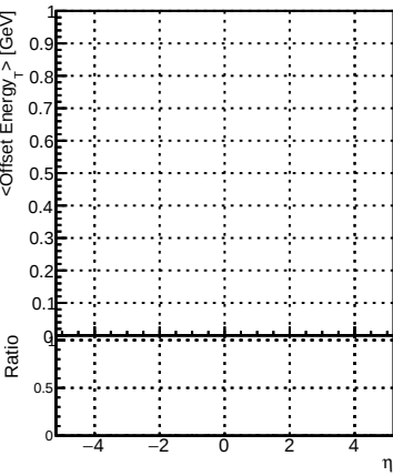
p_offset_eta_npv26_hfh
