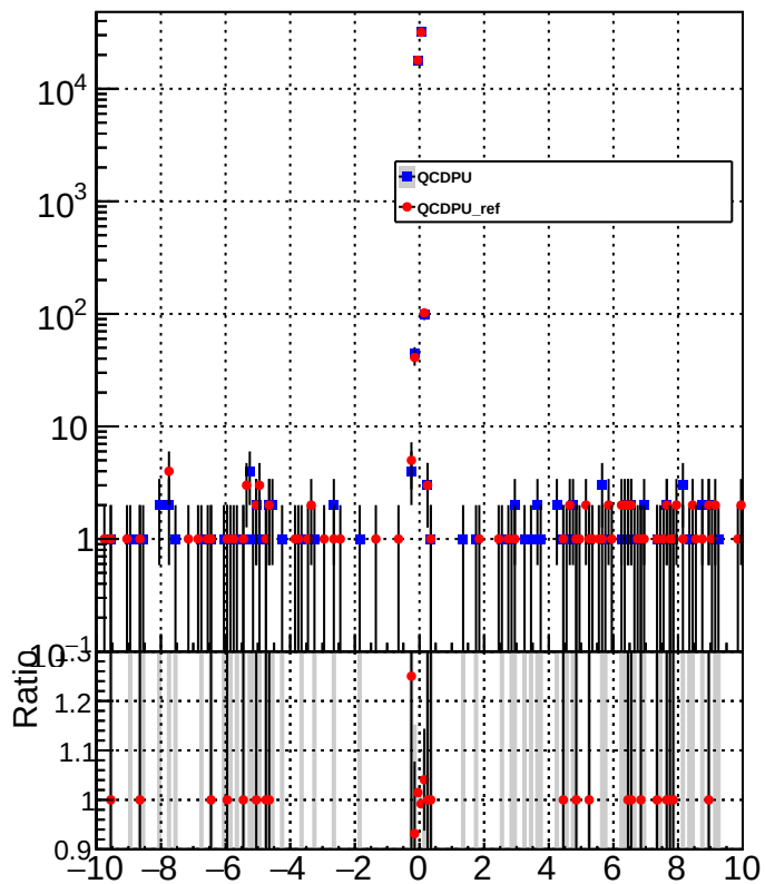
METUnc_MuonEnUp
