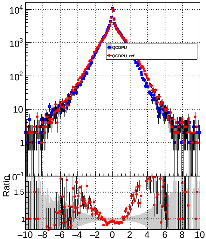
METUnc_UnclusteredEnDown
