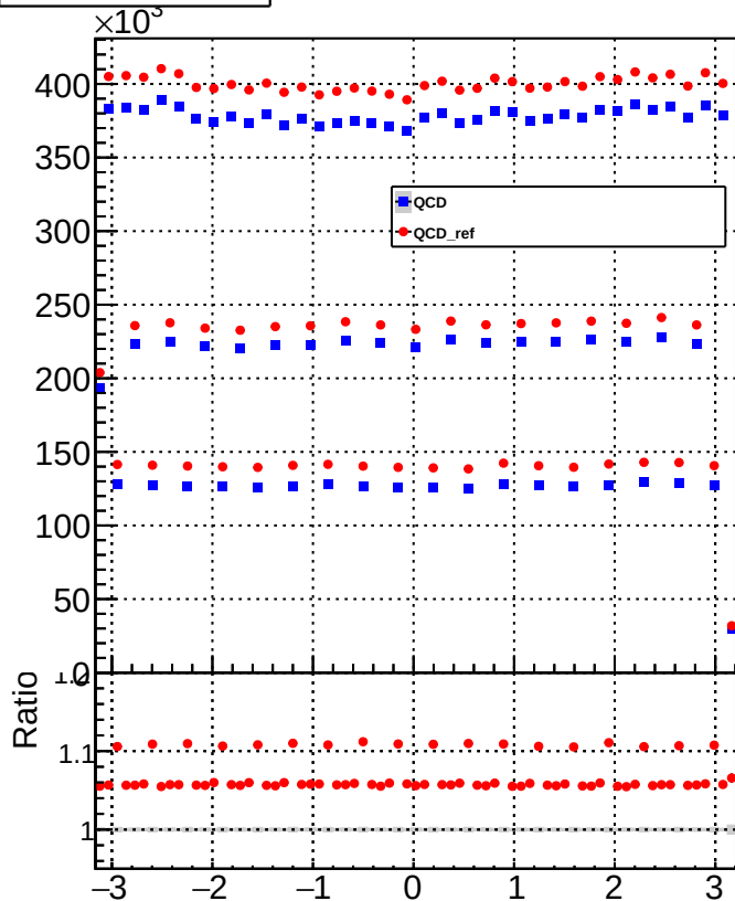
AllCandidatePhi
