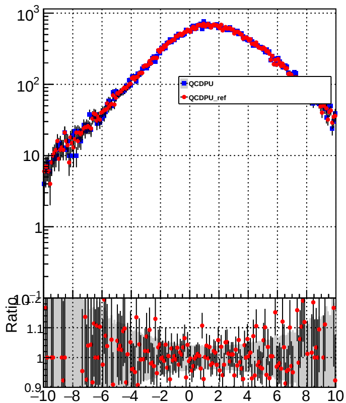
METUnc_JetEnDown
