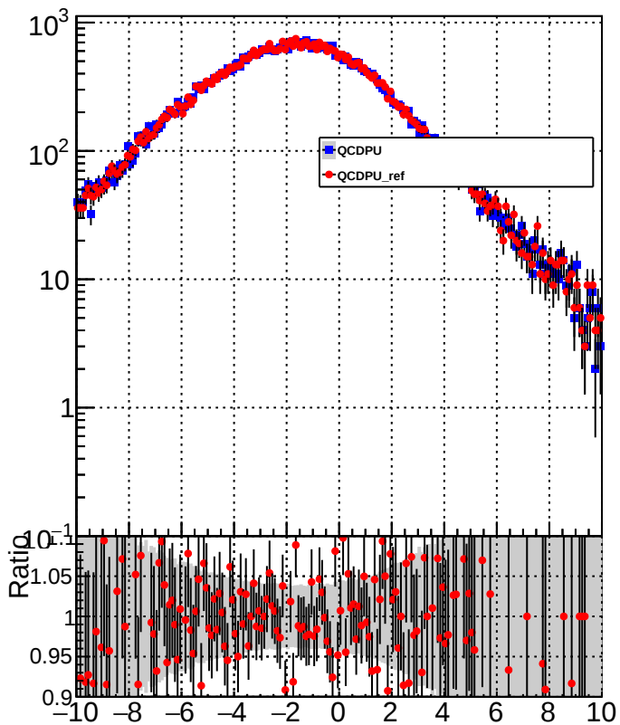
METUnc_JetEnUp
