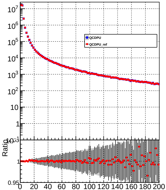
AllCandidatePtMid
