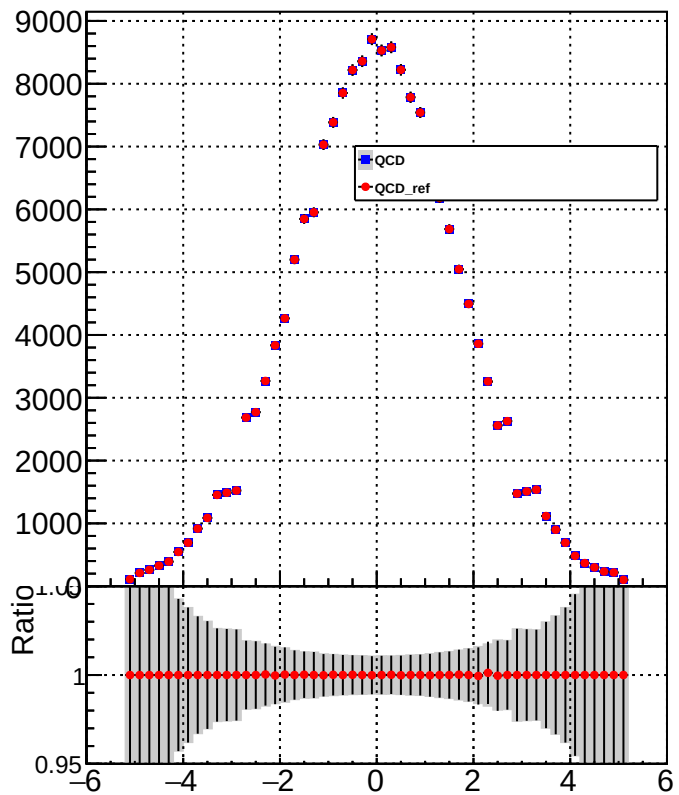
CorrJetEta Pt>20
